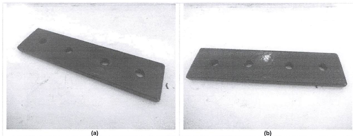
Figura 7 (a) e (b): Macrofoto evidenciando amostra após 648 h de exposição à névoa salina.
