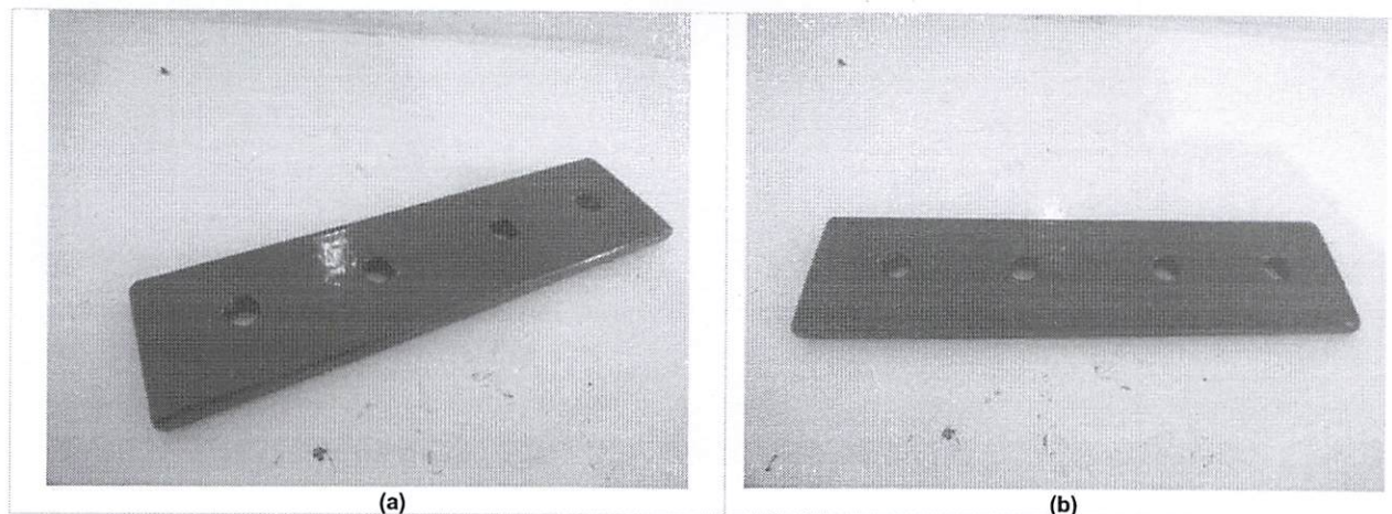
Figura 12 (a) e (b): Macrofoto evidenciando amostra após 1152 h de exposição à névoa salina.
