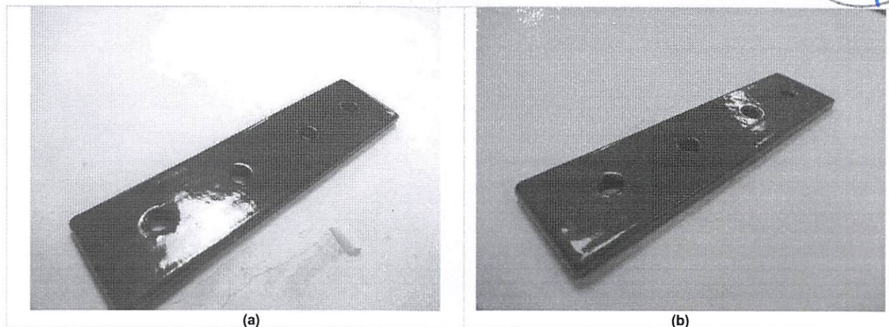
Figura 14 (a) e (b): Macrofoto evidenciando amostra após 1368 h de exposição à névoa salina.
