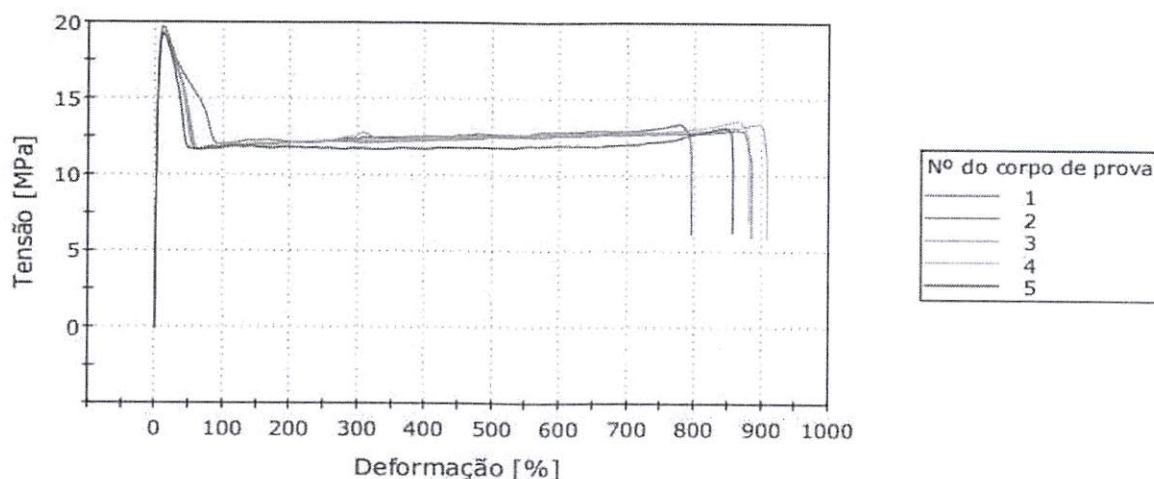
Figura 2 - Curvas Tensão x Deformação da amostra AFK243823.
