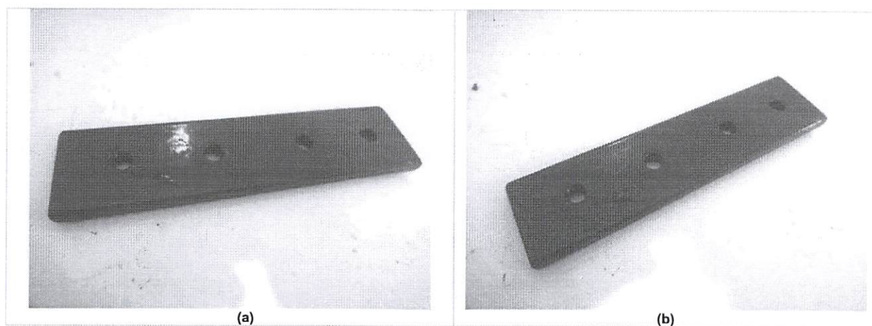
Figura 11 (a) e (b): Macrofoto evidenciando amostra após 1008 h de exposição à névoa salina.
