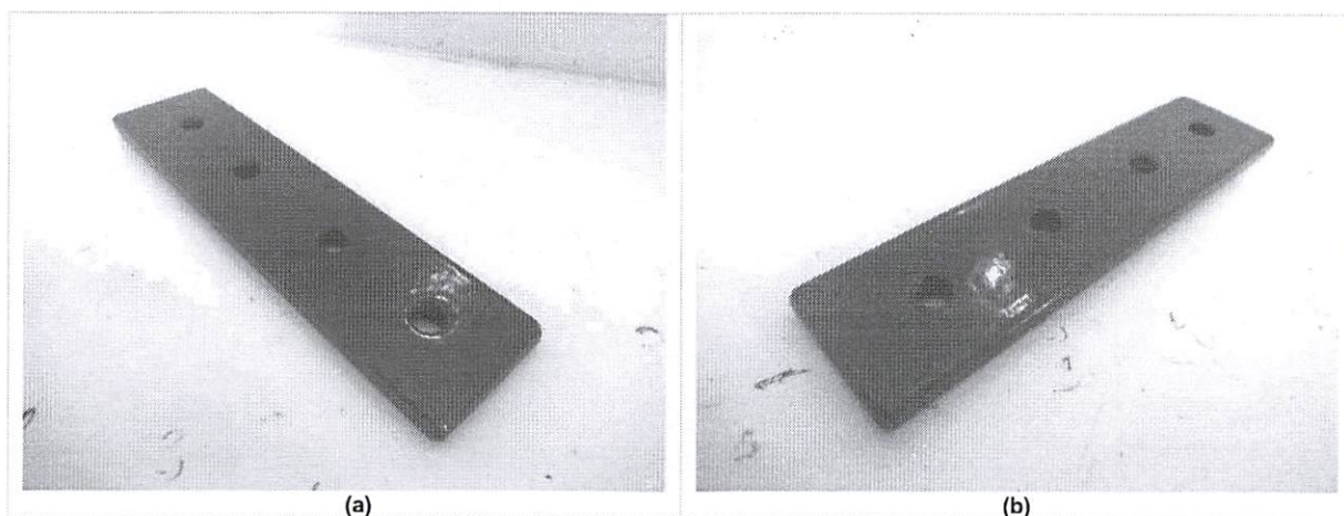
Figura 9 (a) e (b): Macrofoto evidenciando amostra após 864 h de exposição à névoa salina.
