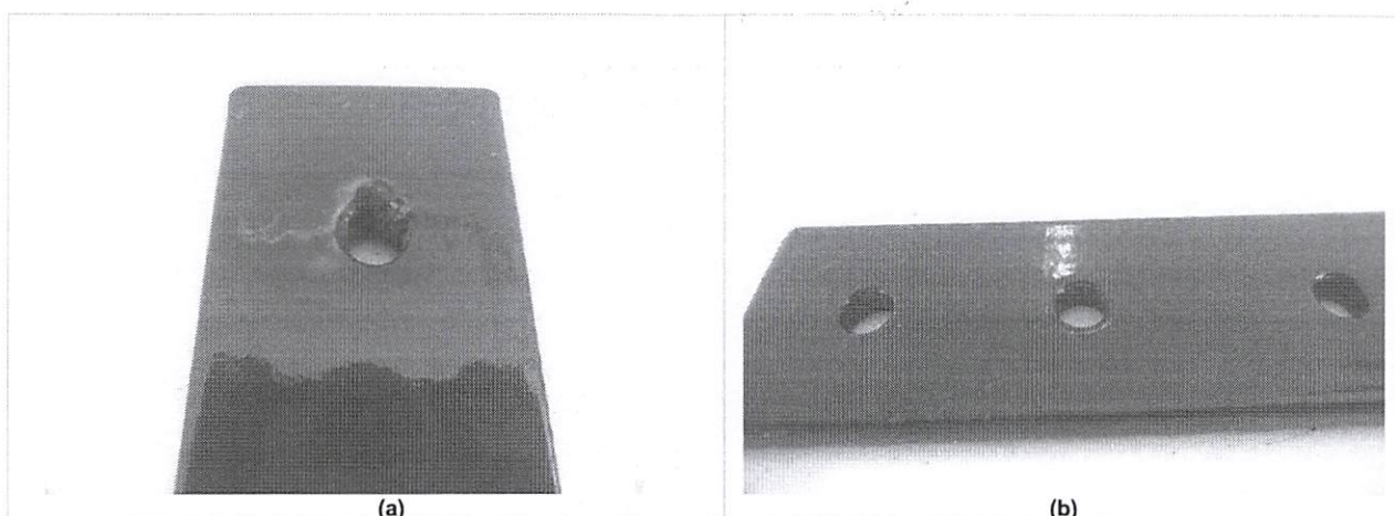
Figura 26 (a) e (b): Macrofoto evidenciando amostra após 2736 h de exposição à névoa salina.
