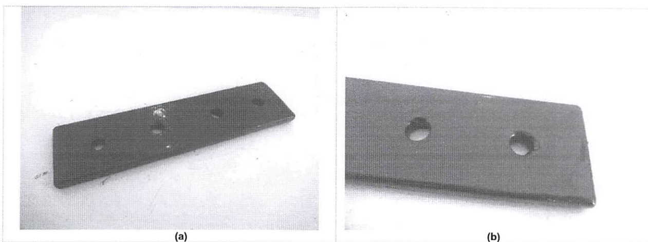
Figura 13 (a) e (b): Macrofoto evidenciando amostra após 1296 h de exposição à névoa salina.
