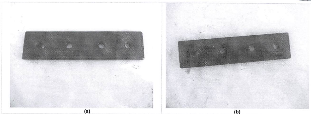
Figura 22 (a) e (b): Macrofoto evidenciando amostra após 2448 h de exposição à névoa salina.
