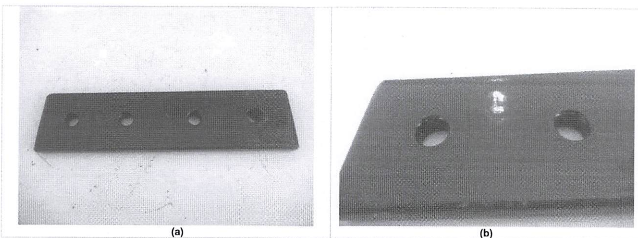
Figura 23 (a) e (b): Macrofoto evidenciando amostra após 2520 h de exposição à névoa salina.
