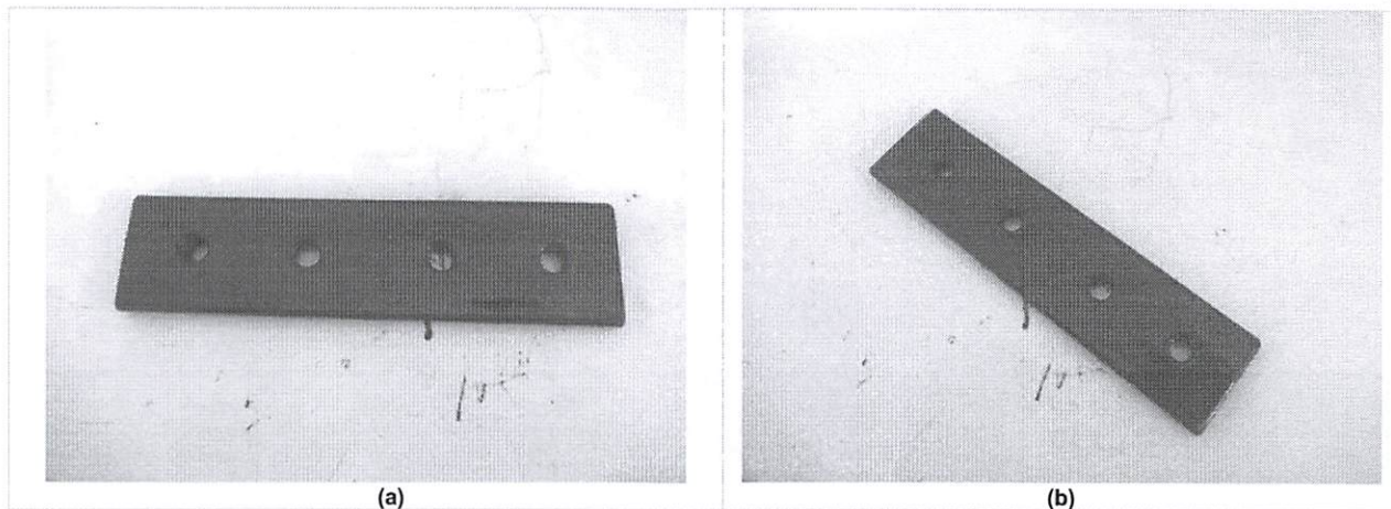
Figura 16 (a) e (b): Macrofoto evidenciando amostra após 1512 h de exposição à névoa salina.
