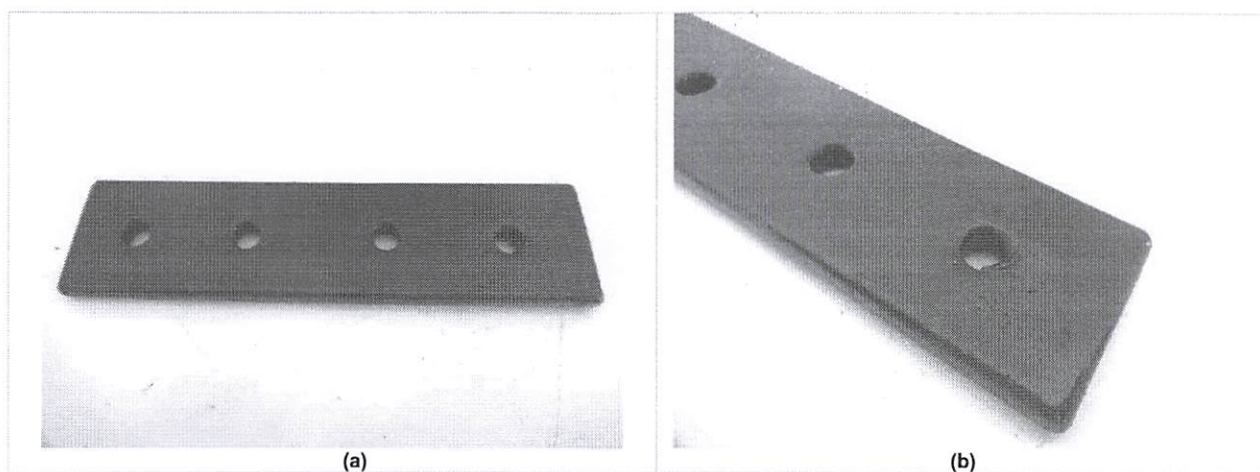
Figura 15 (a) e (b): Macrofoto evidenciando amostra após 1440 h de exposição à névoa salina.
