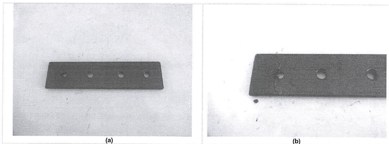
Figura 21 (a) e (b): Macrofoto evidenciando amostra após 2280 h de exposição à névoa salina.
