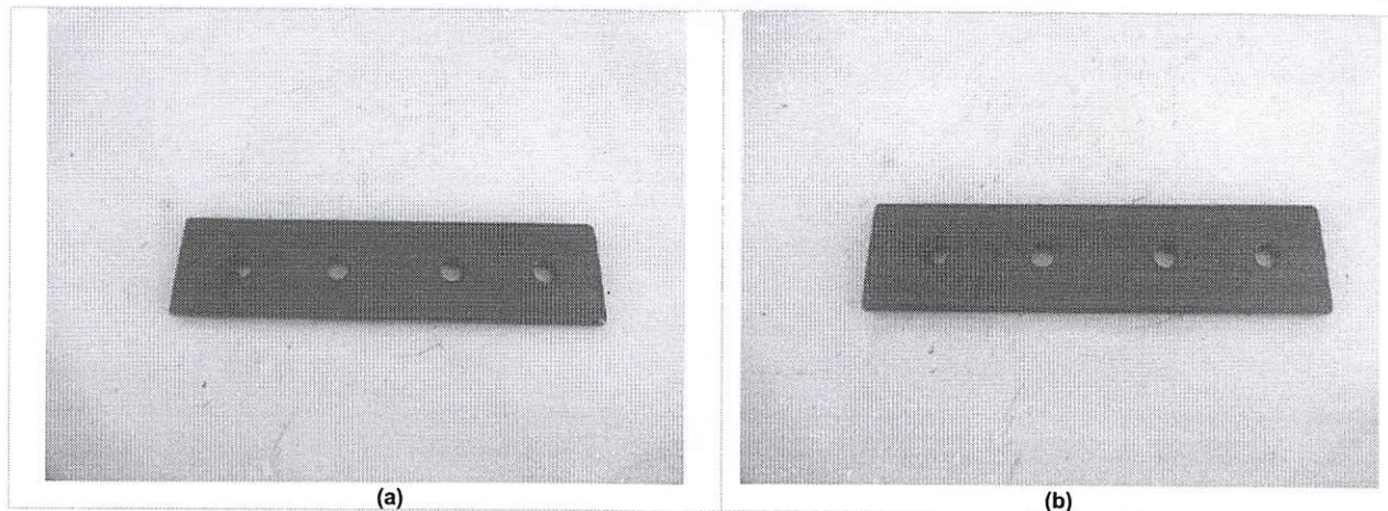
Figura 20 (a) e (b): Macrofoto evidenciando amostra após 2160 h de exposição à névoa salina.
